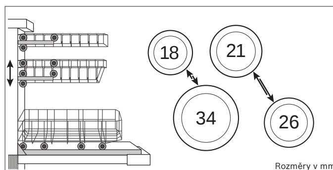
Systém košů s 3. košem Extra Space u myček vysokých 86,5 cm (o 5 cm vyšší myčka nádobí poskytuje prostor navíc pro vysoké nádobí v dolním koši)
